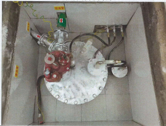
双层油罐和双层管道渗漏检测报警仪
