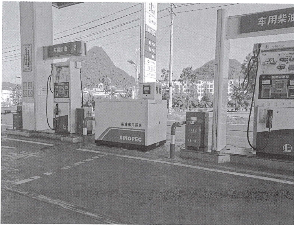
尿素加注机
