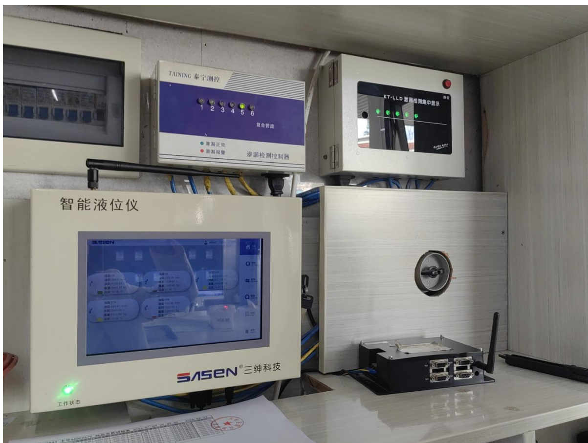
液位仪、渗漏检测仪、紧急切断
